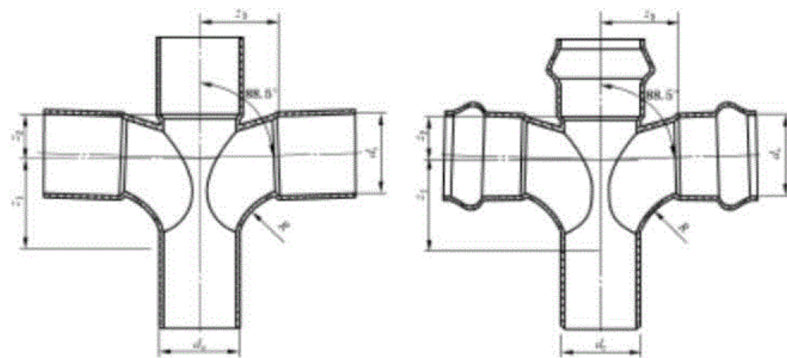
b) 90°带插口正四通示意图
