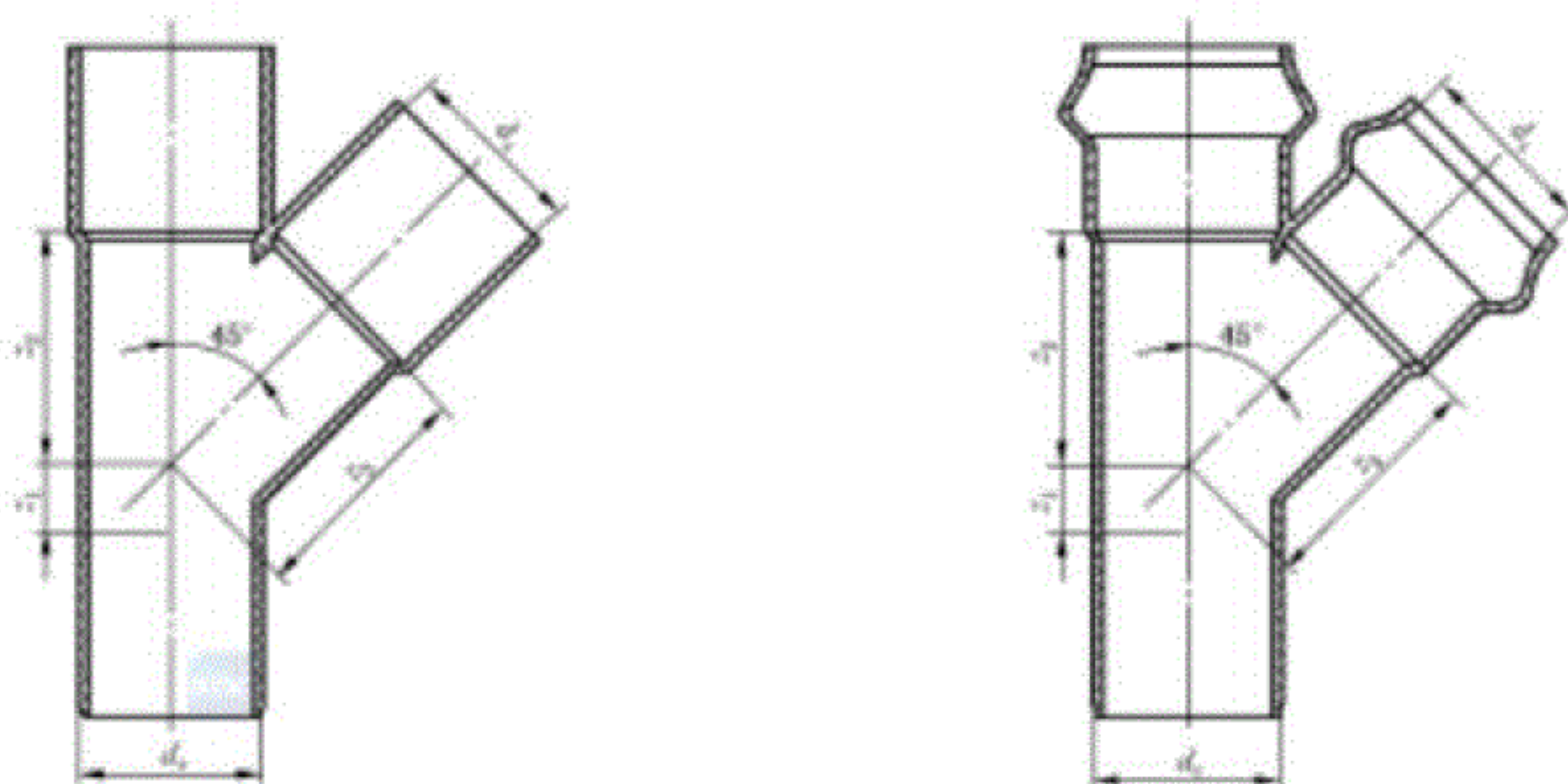
b) 45°带插口斜三通示意图
