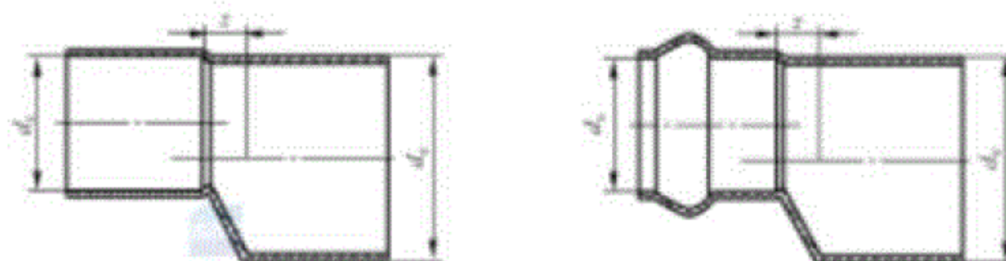
图 B.6 异径示意图
