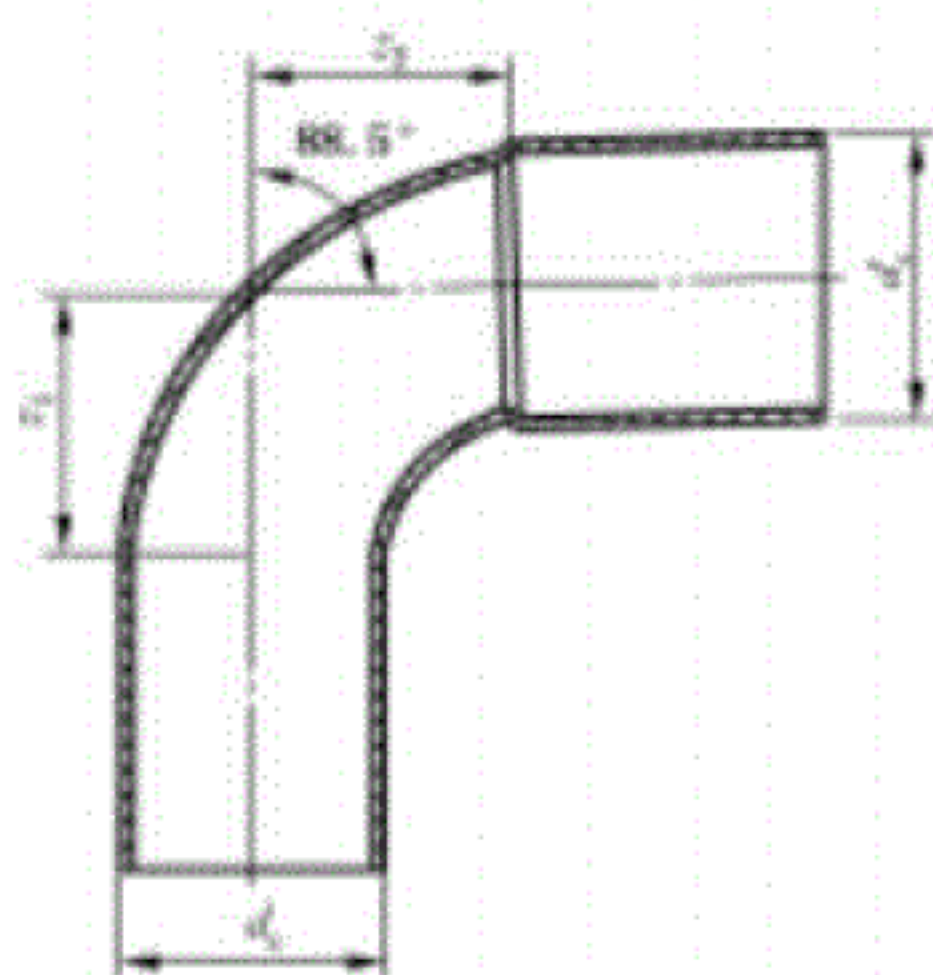
d) 90°带插口弯头示意图
