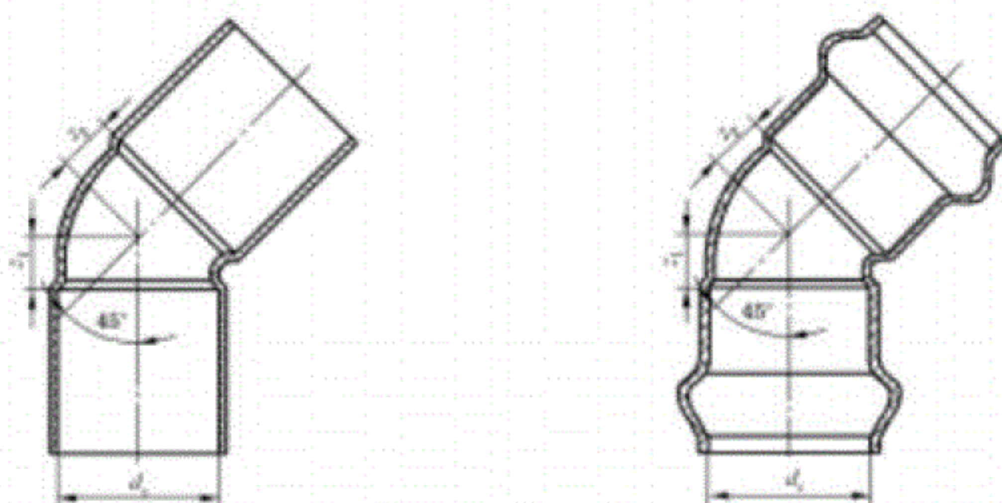
a) 45^\circ 弯头示意图
