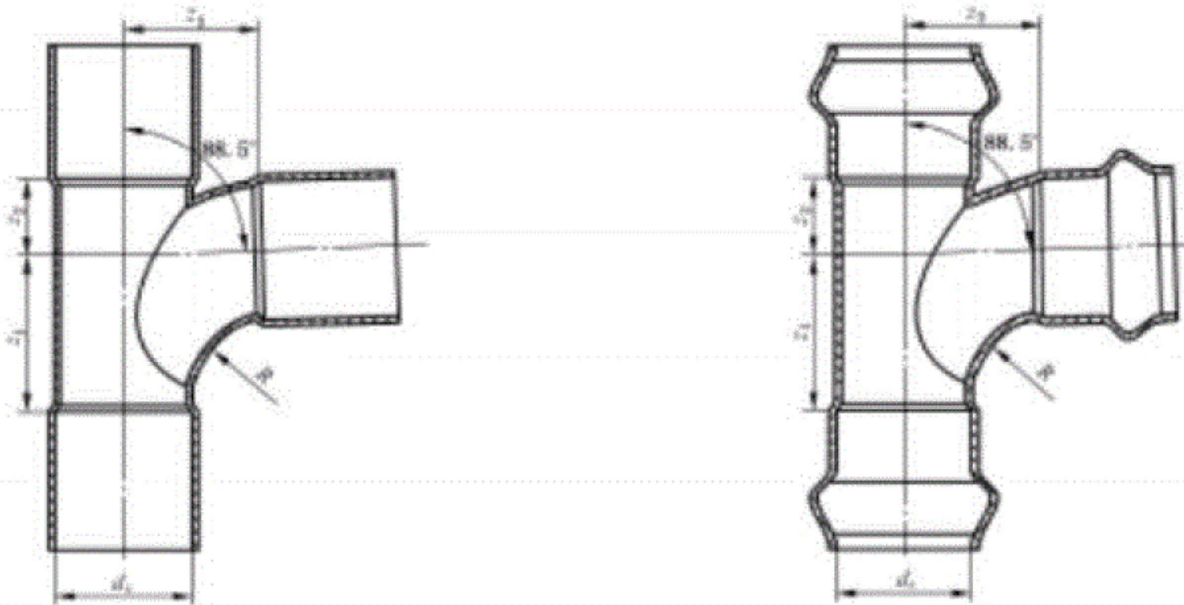
a) 90°顺水三通示意图
