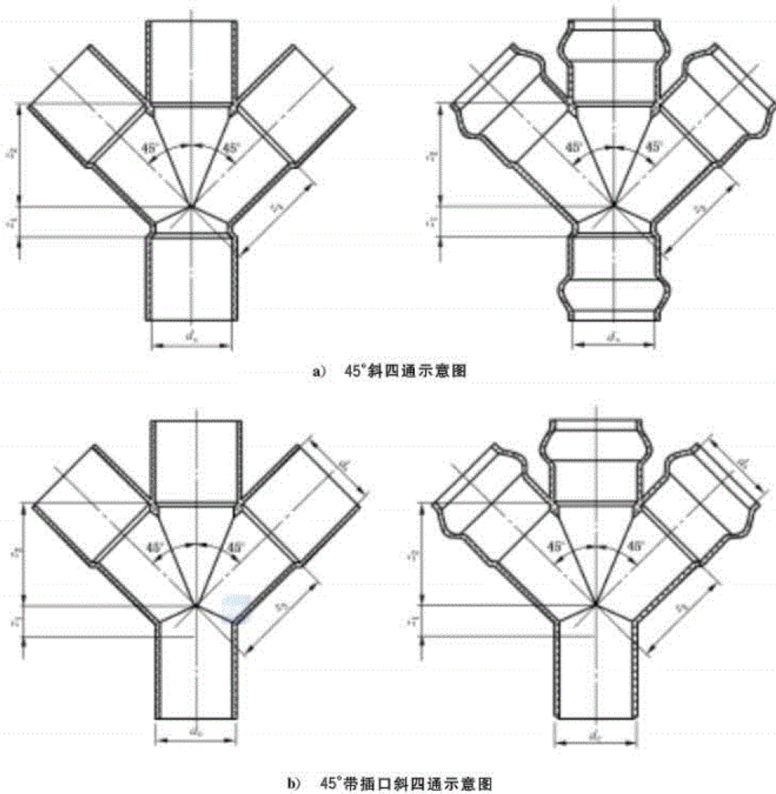
图 B.4 45°四通示意图
