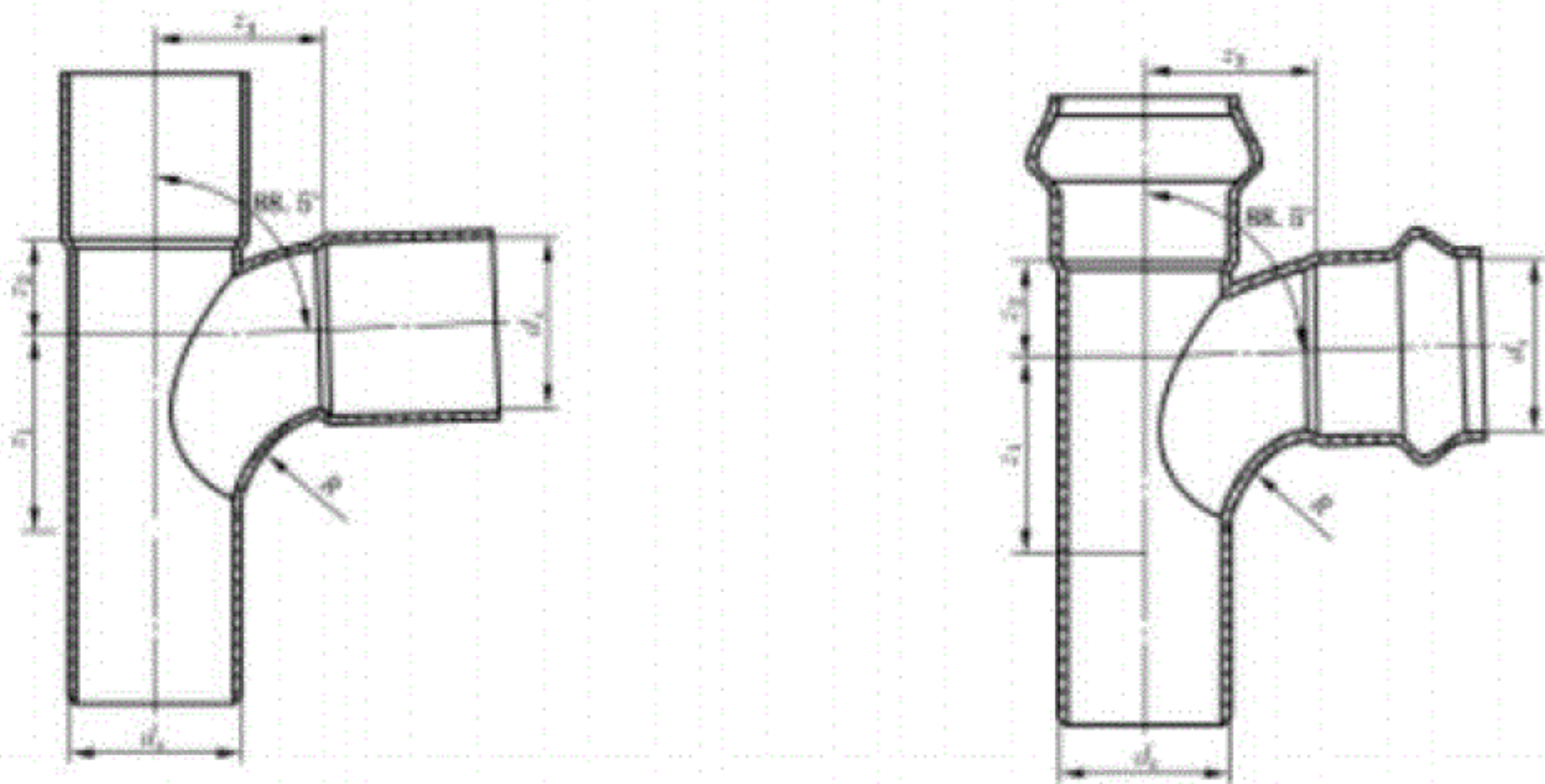
b) 90°带插口顺水三通示意图
