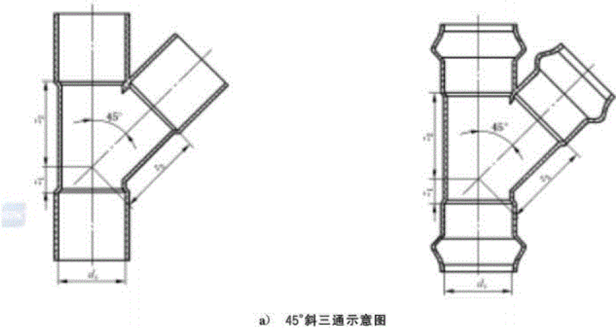
图 B.2 45°三通示意图
